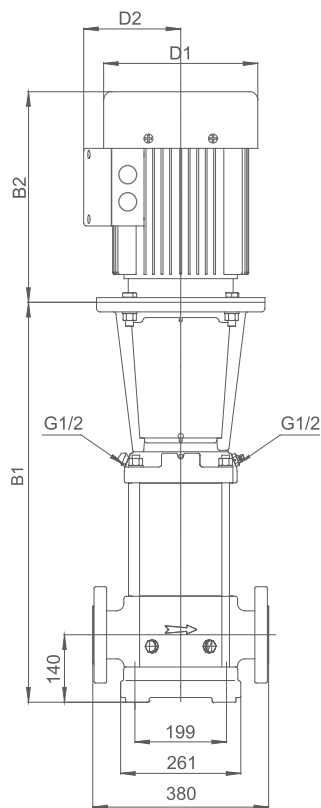
DIN FLANGE
