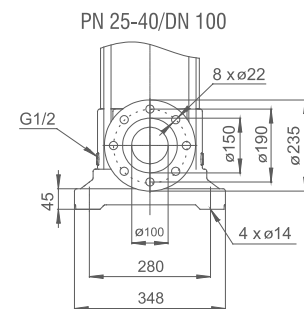
DIN FLANGE / (SS)
