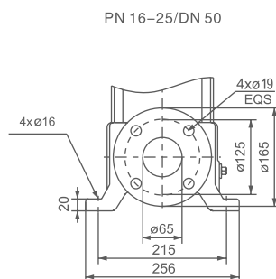
DIN FLANGE PVMP
