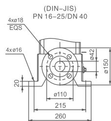
DIN FLANGE
