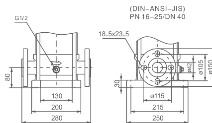
DIN FLANGE (SS)
