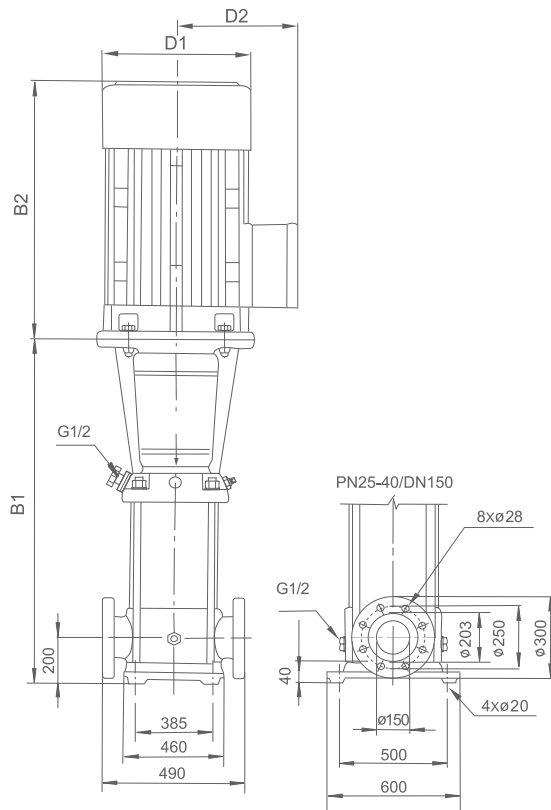
DIN FLANGE / (SS)
