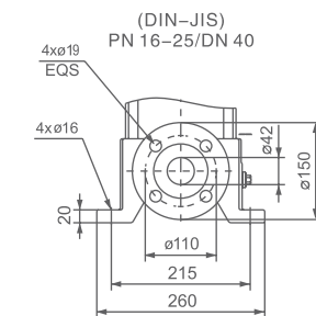
DIN FLANGE
